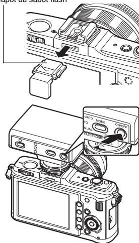
Capot du sabot flash
