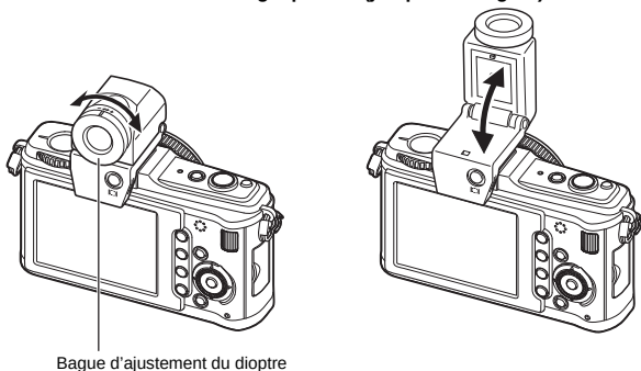
Bague d'ajustement du dioptre
